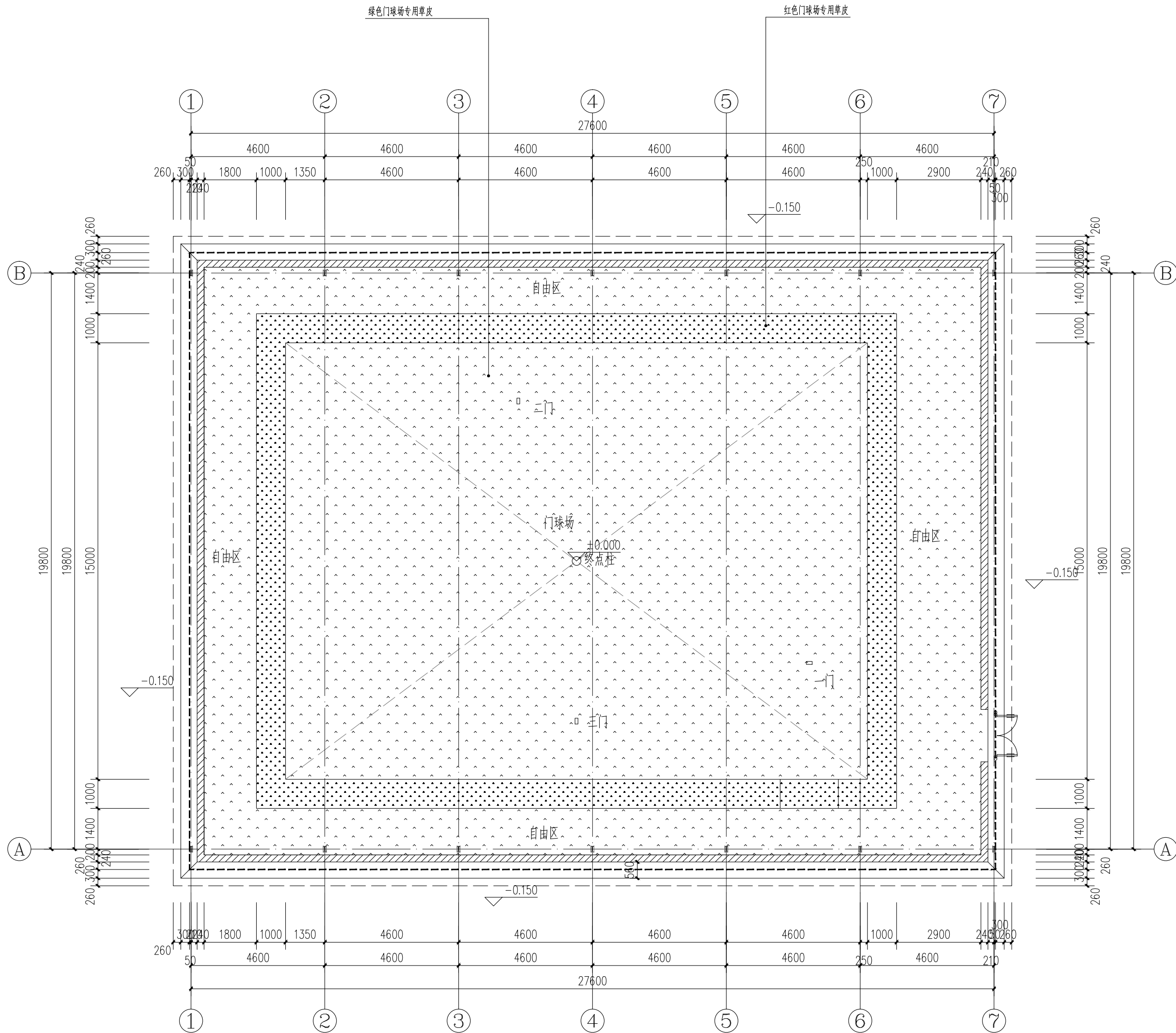
门球场铺装平面图
