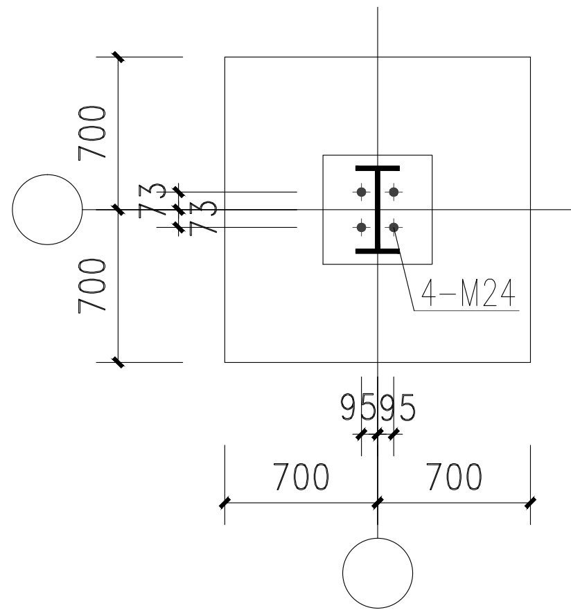
DJ1螺栓定位图
