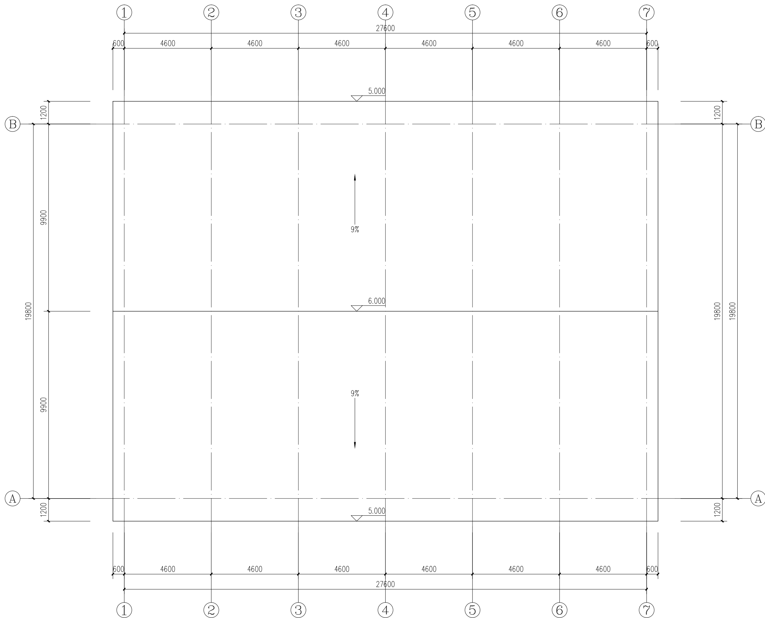
定制电动伸缩遮阳雨棚屋顶平面图
