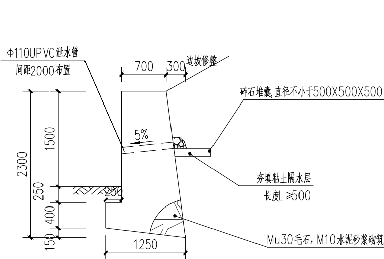
B段挡土墙断面图
