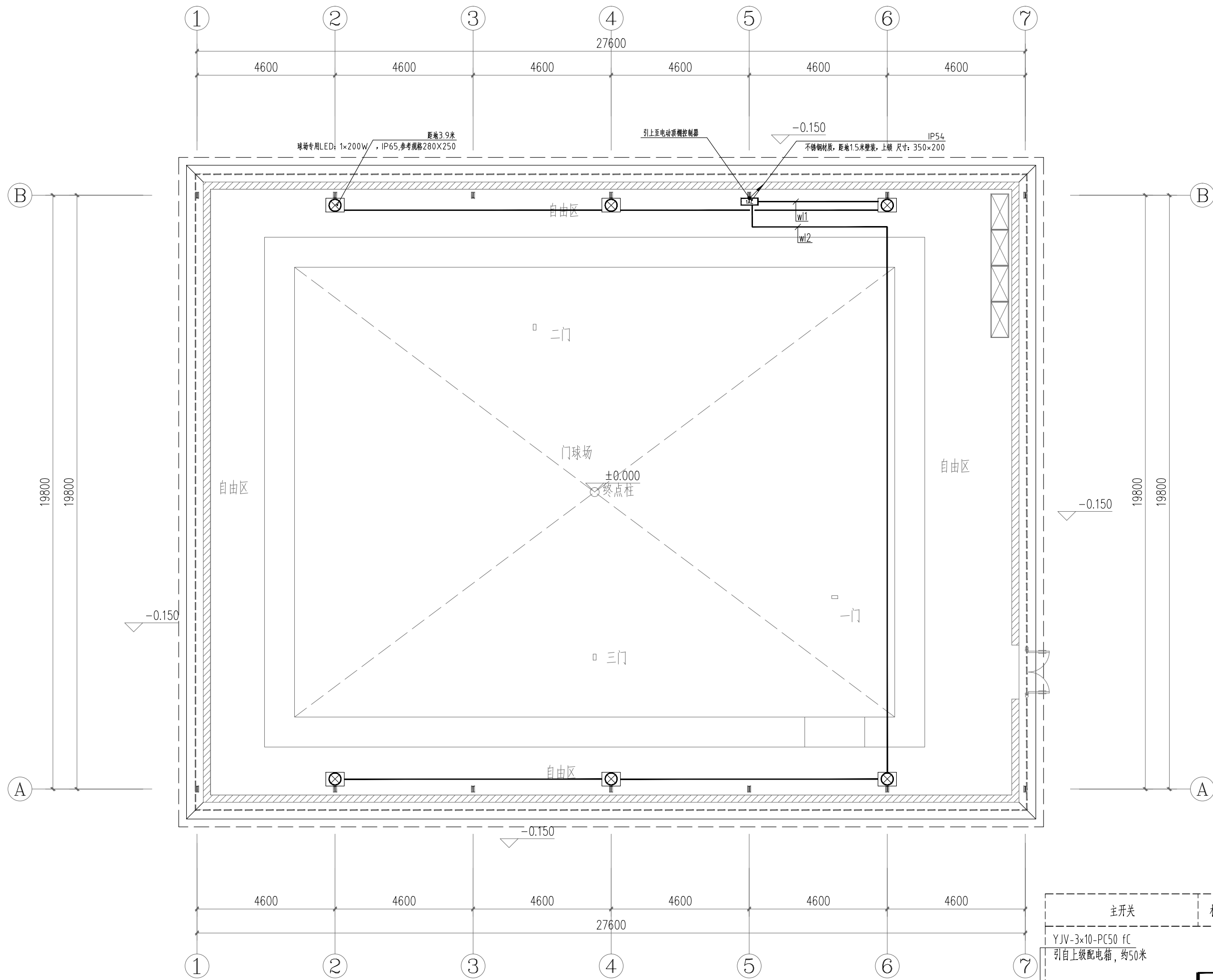
门球场电气平面图
