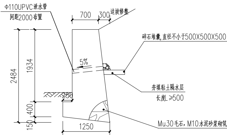
A段挡土墙2-2断面图
