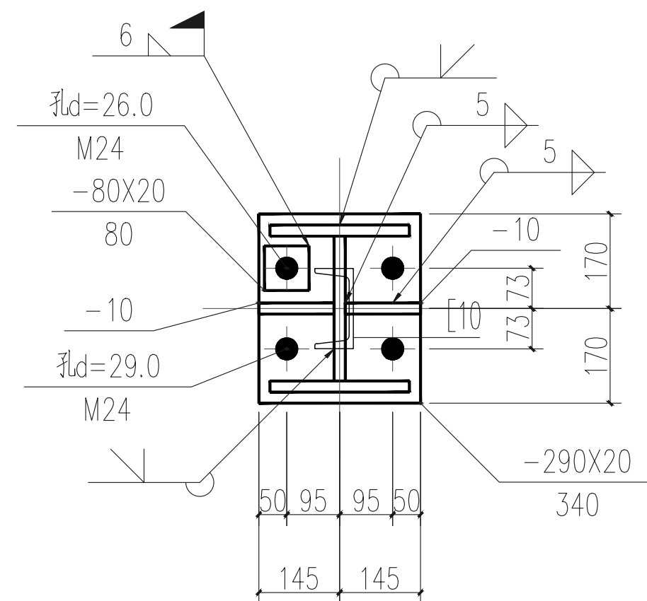
A - A
