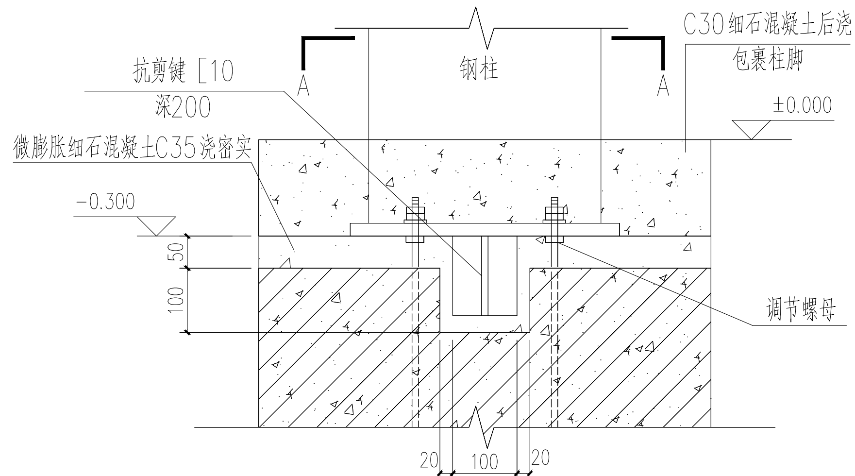
柱脚抗剪键详图
