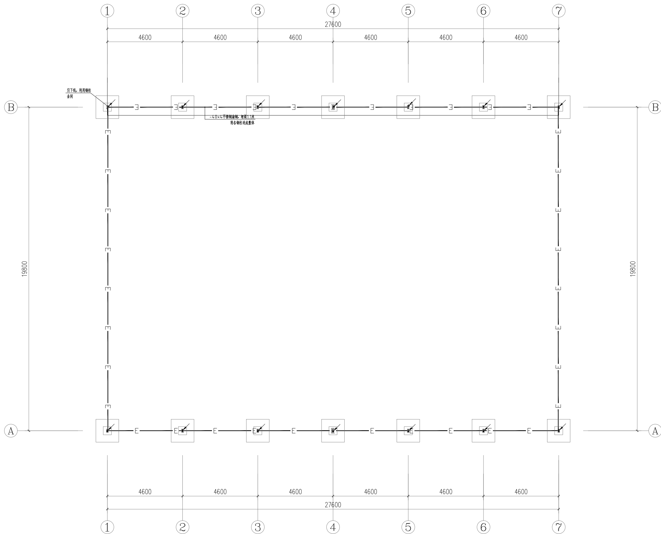
门球场基础接地平面图
