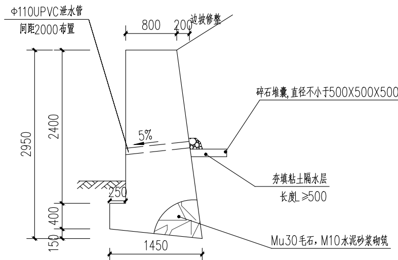
A段挡土墙1-1断面图
