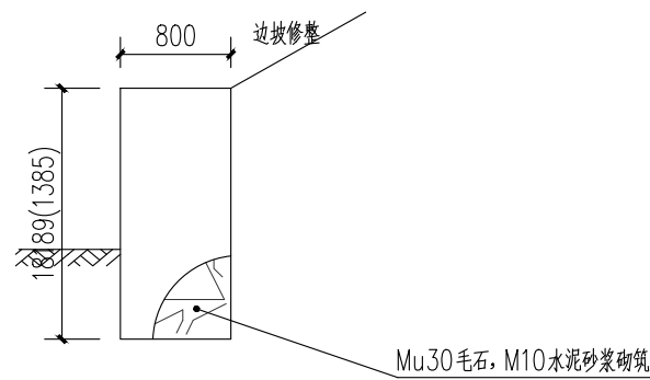
A段挡土墙1-1断面图
